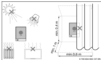
Afb. 4 Montageplaats thermostaat
