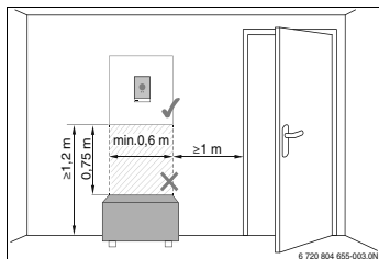
Afb. 3 Montageplaats thermostaat - vrije ruimte
