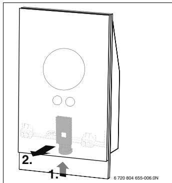
Afb. 7 Demontage thermostaat
