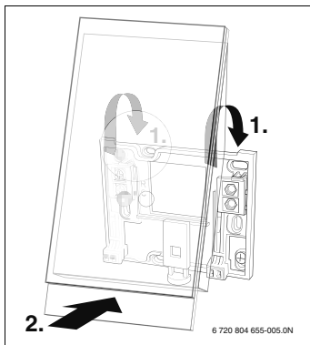
Afb. 6 Monteren thermostaat
