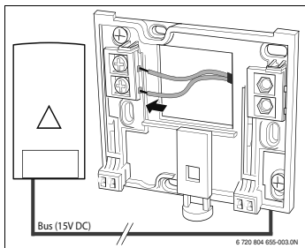
Afb. 5 Aansluiten grondplaat
